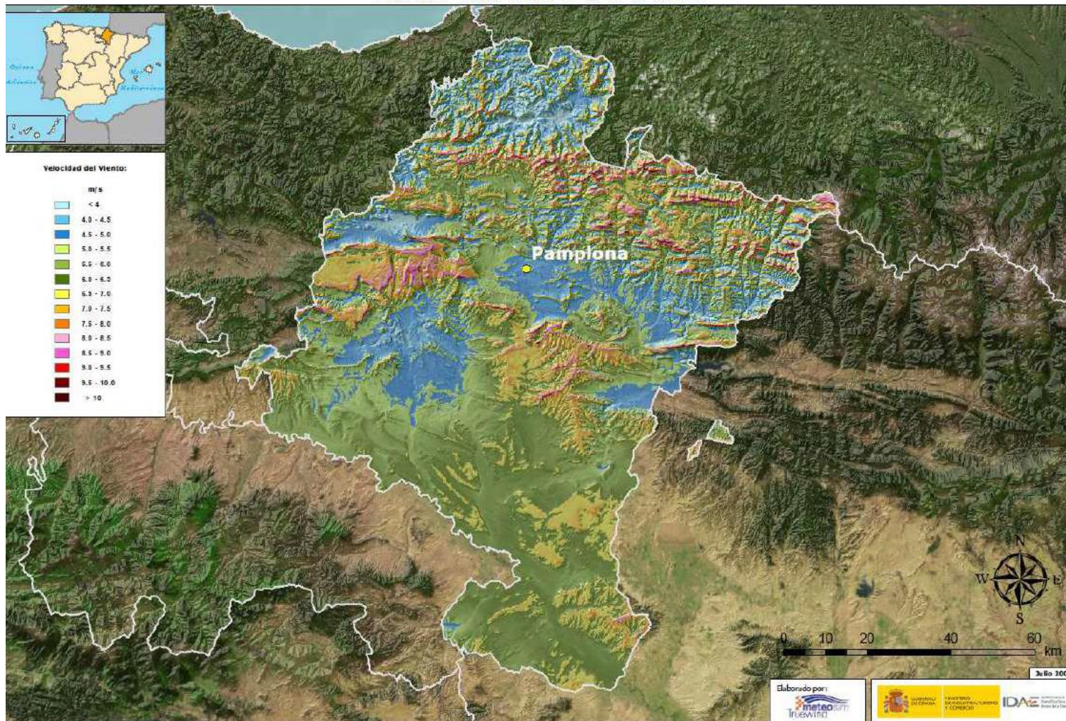
Figura 3-2 Velocidad media anual a 80 metros de altura
