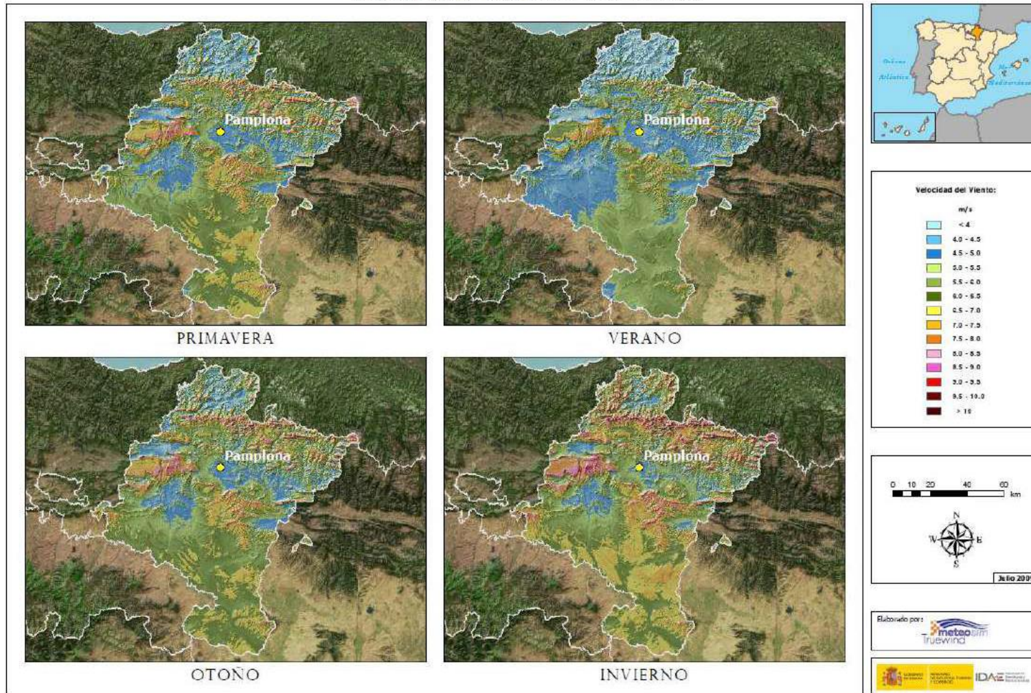
Figura 3-3 Velocidad media estacional a 80 metros de altura
