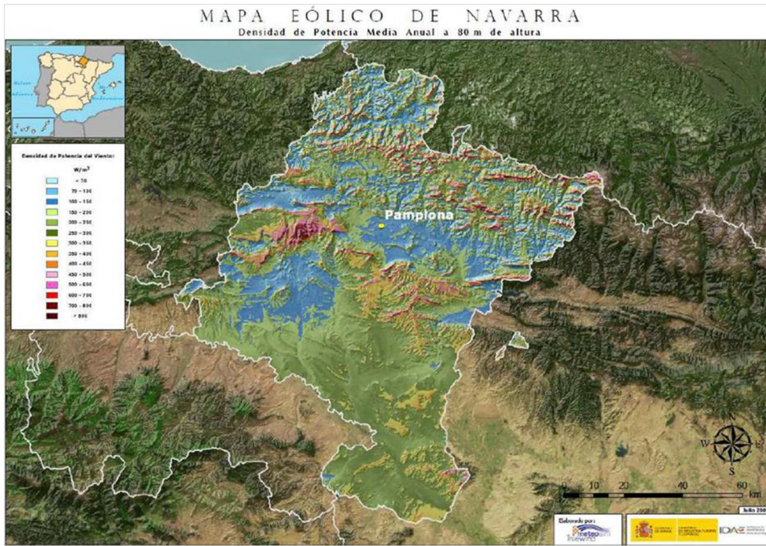
Figura 3-1 Densidad de potencia media anual a 80 metros de altura
