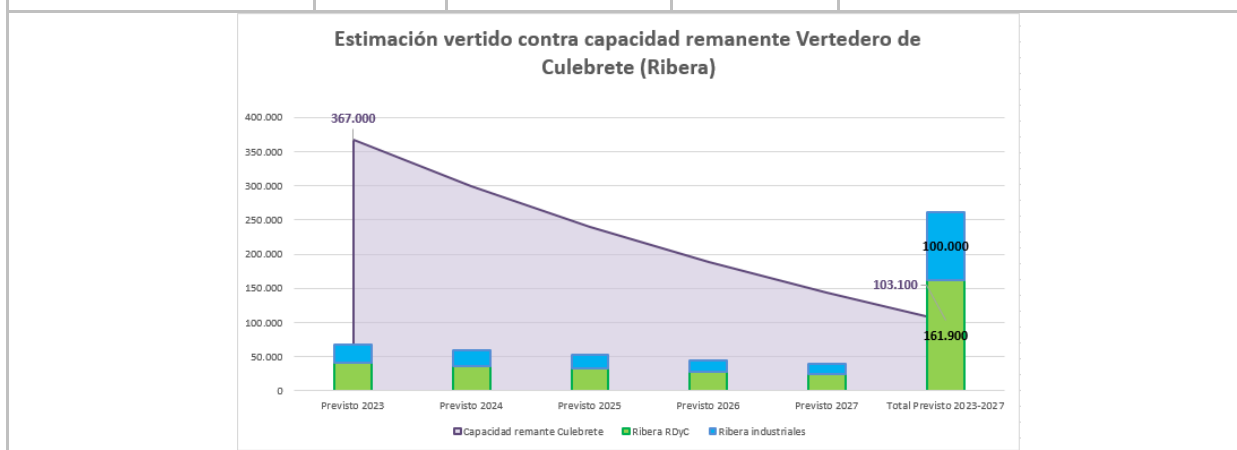
Imagen 9. Estimación vertido contra capacidad remanente vertedero del Culebrete (Mancomunidad de la Ribera). Fuente: elaboración propia (GAN-NIK)
